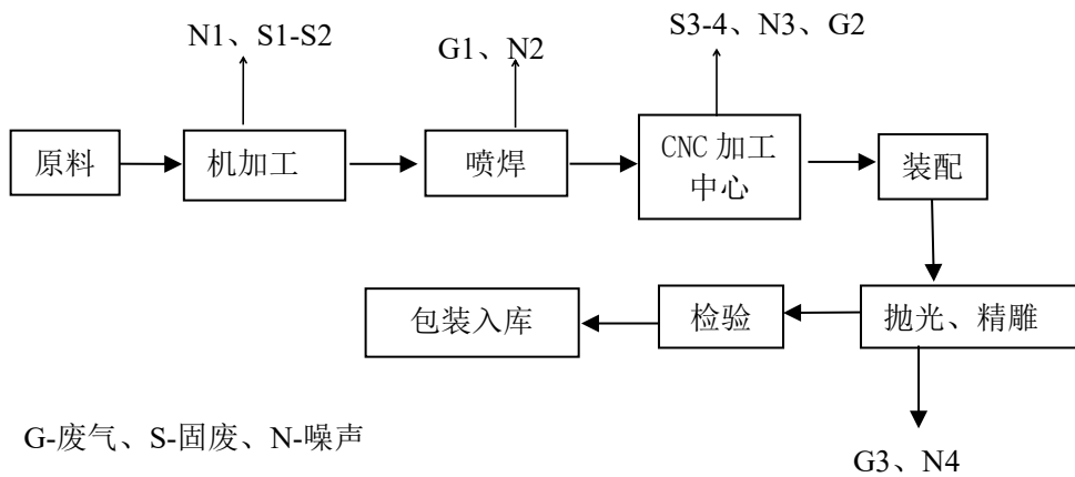
图 2-2 工艺流程图
