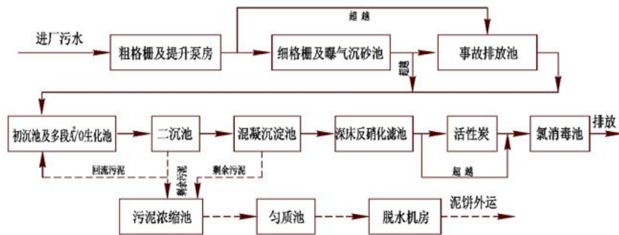
图 4.2-1 常熟市城东水质净化厂废水处理工艺流程图
