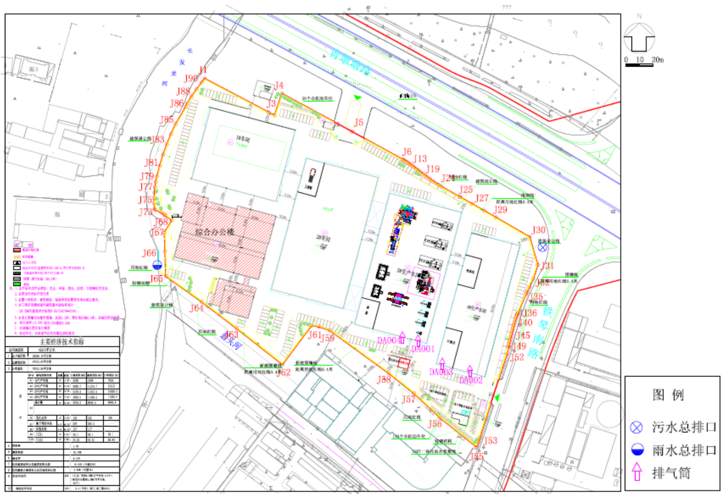
附图3.1 厂区平面布置图
