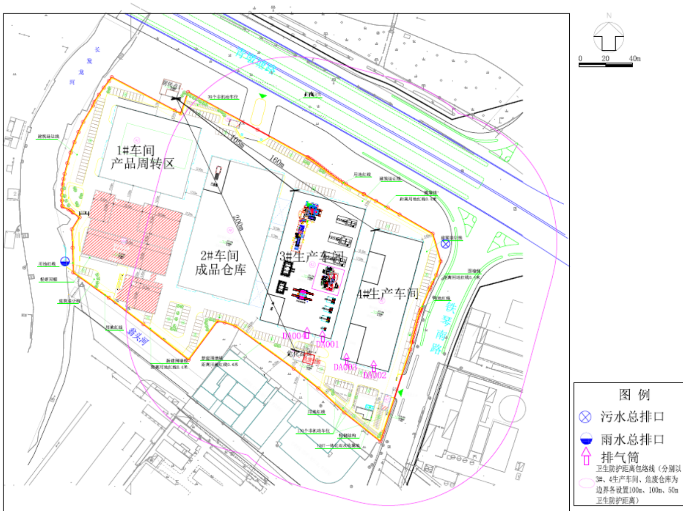
图6.1 本项目卫生防护距离包络图
