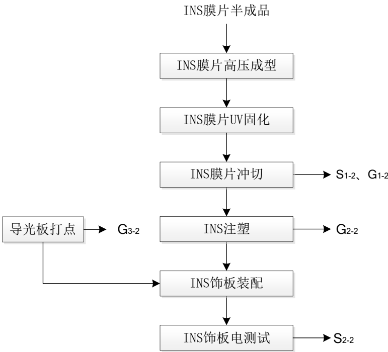
图 2-4 INS 内饰件生产工艺流程图
