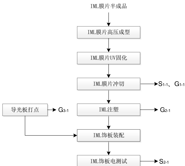
图 2-3 IML 内饰件生产工艺流程图
