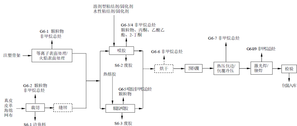
图 2-7 现有项目门板、副/仪表板生产工艺流程及产污环节图
