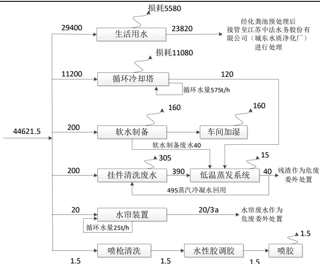
图 2-2 扩建后全厂水平衡图 (t/a)
