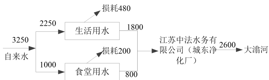
图 2-1 本项目水平衡图 (t/a)
